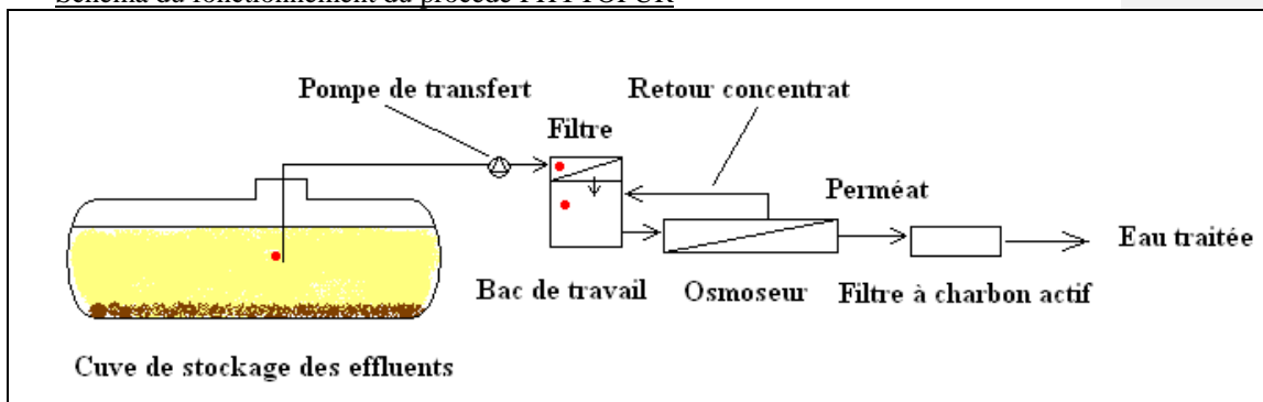
Schéma du fonctionnement du procédé PHYTOPUR®
